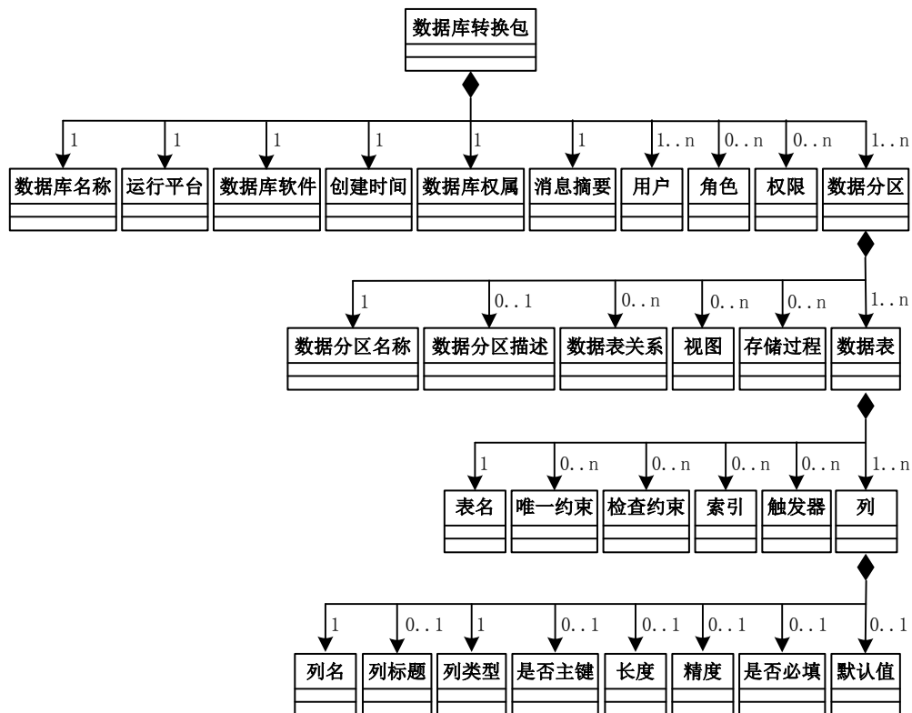
图 2 数据库元数据的层次模型
