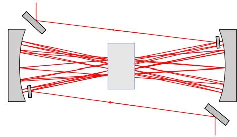
图 1 基于 Herriott 型多通结构的块材料展宽器示意图 Fig. 1. Schematic diagram of block material stretcher based on Herriott.
