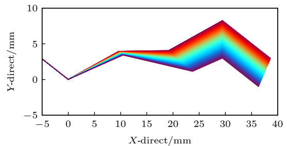
图 4 棱栅对内部光线追迹图
