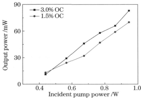
图 3 激光输出功率随入射功率的变化曲线
