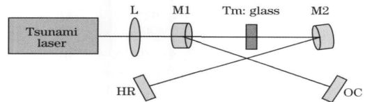
图 2 掺杂 \text{Tm}_2\text{O}_3 的 FGe 玻璃激光实验装置图 Fig. 2 Experimental setup of the \text{Tm}_2\text{O}_3 doped FGe glass laser
