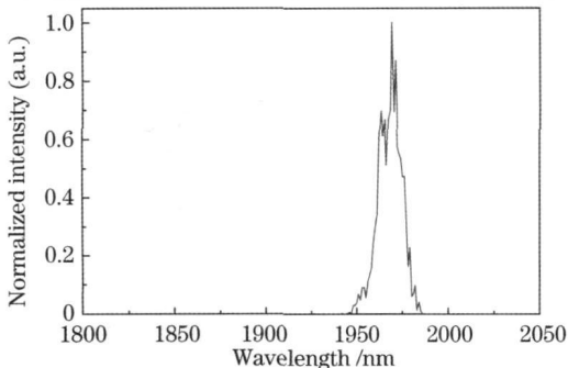
图 4 掺杂 \text{Tm}_2\text{O}_3 的 FGe 玻璃激光输出的光谱图
