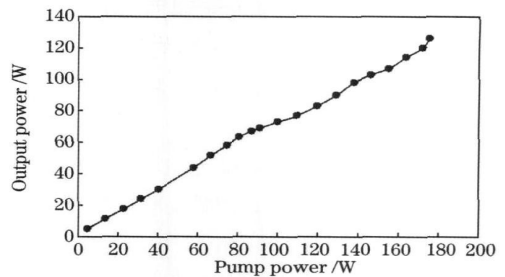
图 1 激光功率随抽运功率的变化曲线
