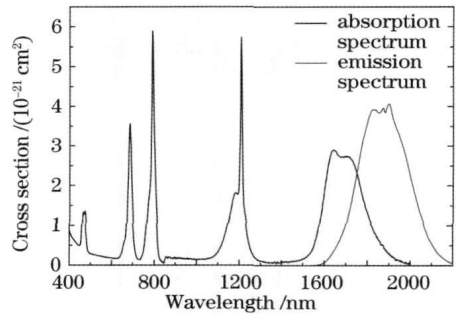
图 1 掺杂 \text{Tm}_2\text{O}_3 的 FGe 玻璃的吸收截面和发射截面曲线
