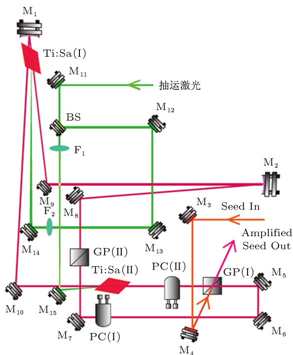
图 1 环形长腔再生放大器光路布局图(图中 M_1, M_2 为曲率半径为 4 m 的 700—900 nm 宽带凹面镜, M_3—M_{10} 为 700—900 nm 45° 全反的宽带平面反射镜, M_{11}—M_{15} 为 45° 532 nm 全反镜, F_1, F_2 为焦距为 1000 mm 的正透镜, BS 为 532 nm 1:1 分束镜, GP(I), GP(II) 为格兰棱镜, PC(I), PC(II) 为普克尔盒, Ti:Sa(I), Ti:Sa(II) 为掺钛蓝宝石晶体)
