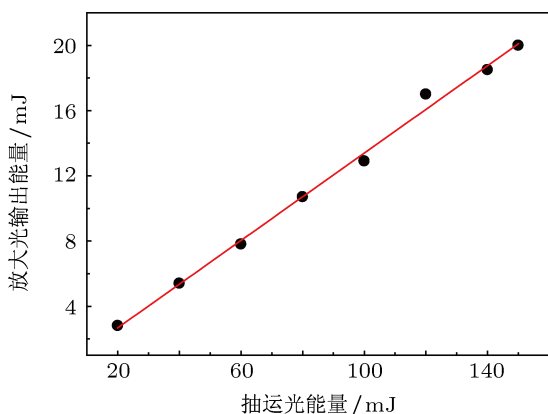
图3 放大激光输出能量随着入射抽运能量的变化(黑点表示实际测量值,红线表示线性拟合结果)
