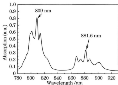
图1 Nd:LGS晶体的吸收光谱
