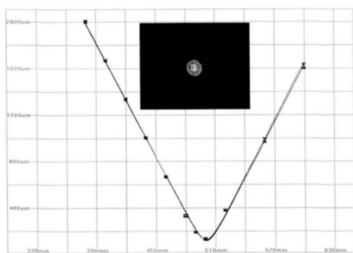
图 4 Nd:LGS 输出激光的 M^2 因子测量结果
