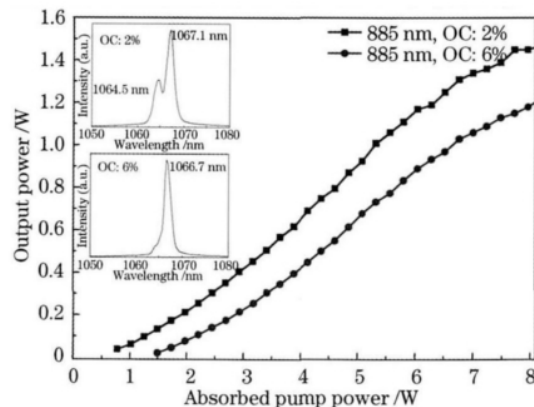
图3 直接抽运下,连续运转时的输入输出功率曲线,插图分别为不同输出耦合率下的激光光谱
