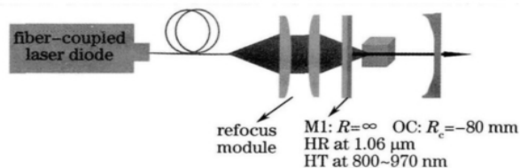
图2 Nd:LGS激光实验装置图
